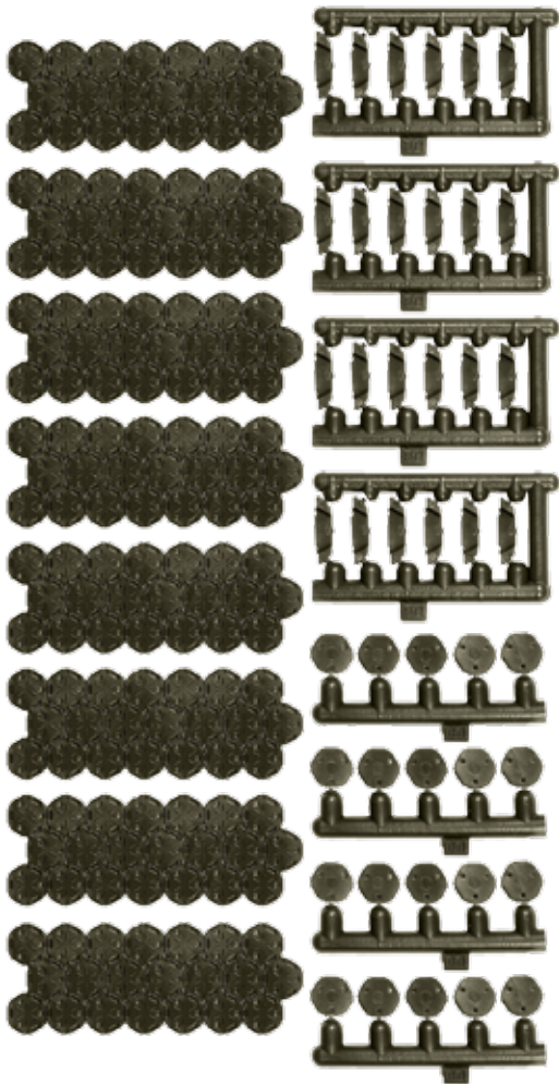
BUNDESWEHR SECHSECKPLATTEN, SECHSECK- PLATTENELEMENTE UND RANDABSCHLÜSSE, BW ENGINEER HEXAGON METAL ELEMENTS, BW 05099
